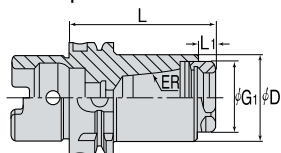
DIN 69893 Форма A
