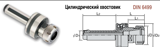
Цилиндрический хвостовик DIN 6499
