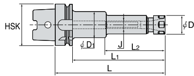
DIN 69893 Форма A
