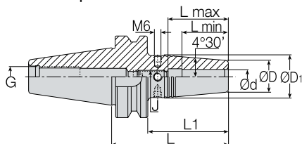
DIN 69871 Форма A/B
