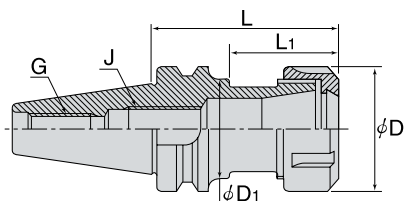
BT MAS 403 Форма A/B
