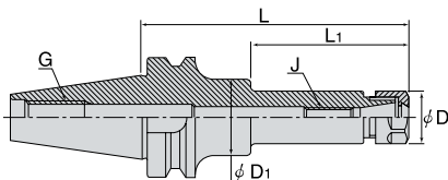
BT MAS 403 Форма A/B
