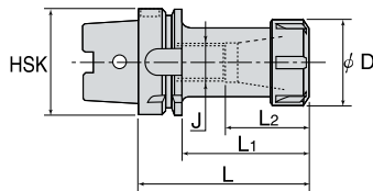
HSK DIN 69893 Форма A
