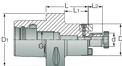
C-АДАПТЕРЫ (ISO 26623-1)
