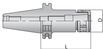
DIN 69871 Форма A/B
