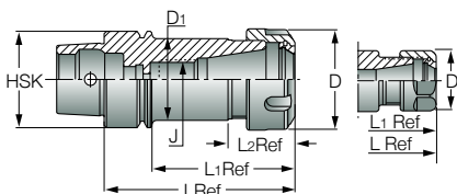
HSK DIN 69896 Форма E
