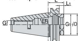
DIN 69871 Форма А/В
