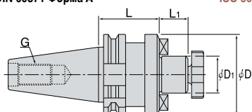
DIN 69871 Форма А
