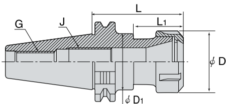
DIN 69871 Форма А/В
